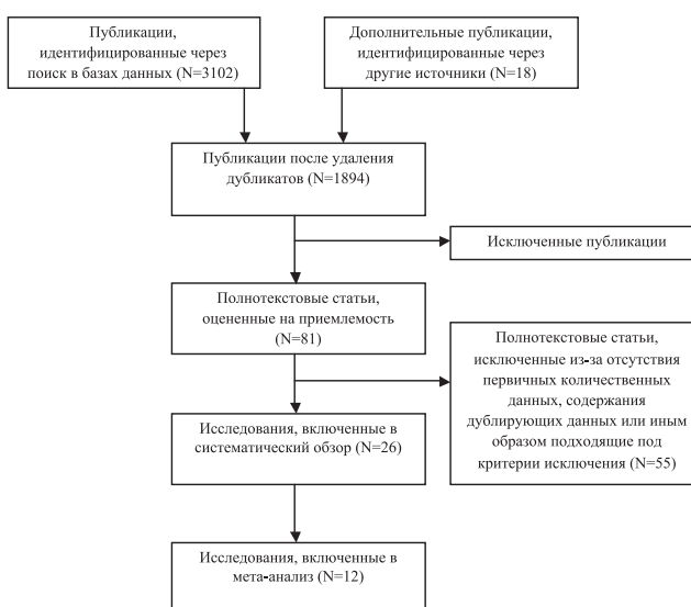
Рис. 1. PRISMA график
